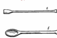
Рис. 1.9. Шпатель (а) и фарфоровая ложка (б)
