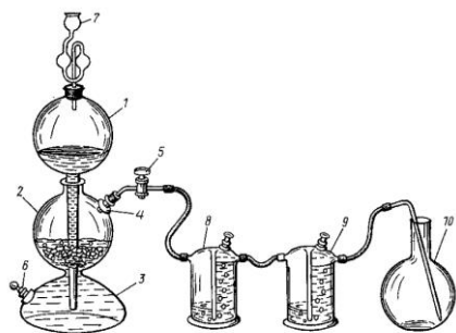
Рис. 1.7. Прибор (аппарат) Киппа. 1, 2, 3 — шарообразные резервуары; 4 — тубус с пробкой и стеклянной трубкой; 5 — кран; 6 — пробка; 7 — предохранительная склянка; 8, 9 — промывалки; 10 — приемник газа
