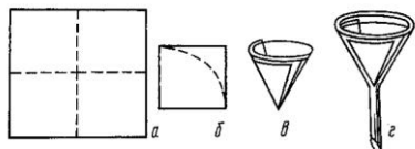
Рис. 1.27. Изготовление простого фильтра: а-е – стадии изготовления; з – фильтр помещен в воронку
