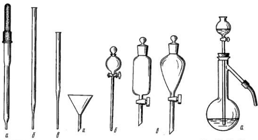
Рис. 1.4. Пипетки: а, б – каменные, в – для отделения жидкости от осадка Рис. 1.5. Химическая (а), капельная (б) и делительная (в) воронки
